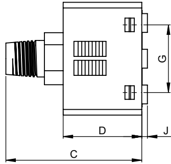
PS1PS-P-1P+K / PS1PS-C-1P+K
