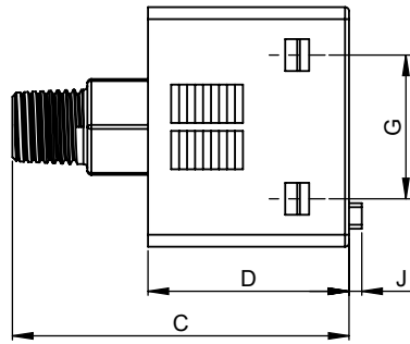
PS1PS-P-2P-420+K / PS1PS-C-2P-420+K
