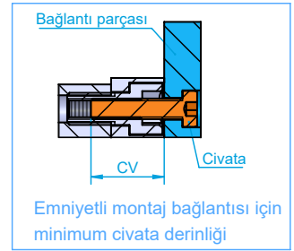
DETAY-D
