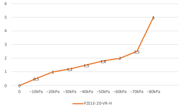
Farklı Vakum Derecelerinde Emme Akış Süresi (-Bar) (s/L)
